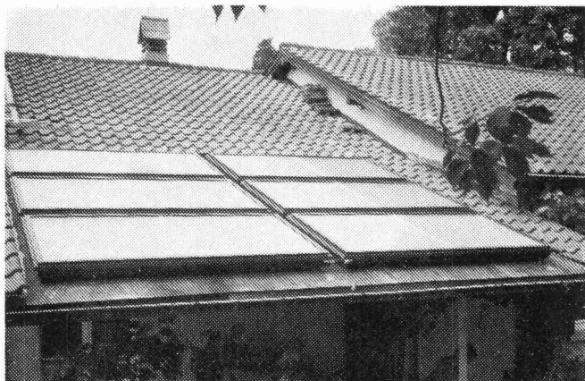
Anlage Erlenbach, 16 m 2 Kollektor, 1500 l Speicher, für Gebrauchswarmwasser und Uebergangsheizung.
