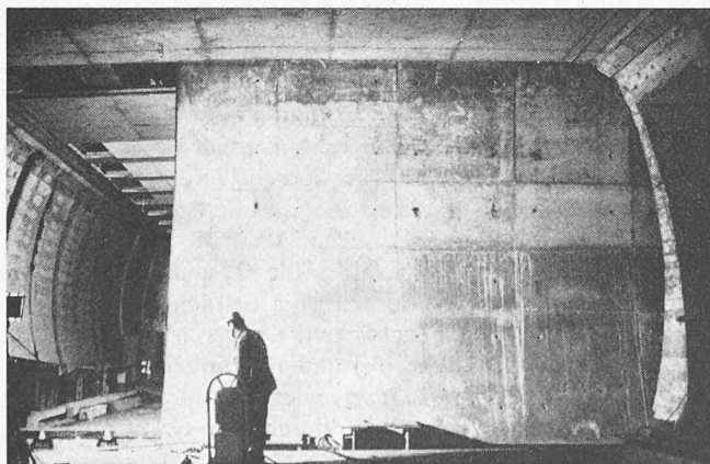
Bild 8. Bogentor im Endzustand, zu zwei Dritteln geschlossen. Am linken Bildrand ist der Zugang zur Torkaverne sichtbar; rechts hinter dem Tor ein Teil der demontablen Tunnelzwischenendecke. In der Bildmitte steht das mobile Hydraulikaggregat für die Torverschiebung
