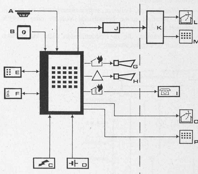
Bild 1. Brandmeldeanlage. Autonome Grundausstattung: links der gestrichelten Linie. Fakultative Zusatzausrüstung: rechts der gestrichelten Linie
