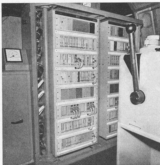
Bild 26. Elektronikblock
