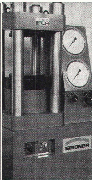
Baustoff-Prüfmaschine
