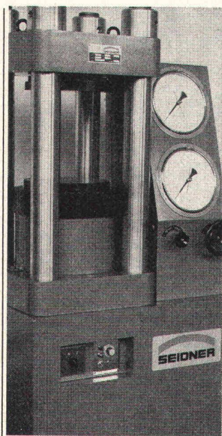
Baustoff-Prüfmaschine
