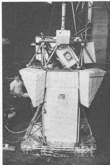
Links: Start bei Sonnenuntergang in Palestine (Texas): Das Helium strömt aus Tankzügen in den Ballon und bläht seine Hülle für den Flug bis in 42 Kilometer Höhe. Von dort aus beobachteten Wissenschaftler mit Hilfe von zwei Röntgenfernrohren die regelmässigen Blitze aus dem Doppelsternsystem Herkules X-1. Rechts: Letzte Tests an der Ballongondel und an den beiden Röntgenfernrohren (Bildmitte).
