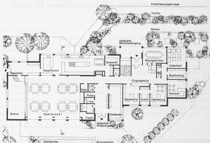
Rechts: Grundriss Erdgeschoss Hauptgebäude 1:450
