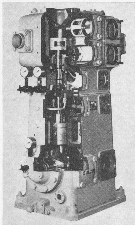
Bild 5. Moderner Labyrinthkolbenkompressor; Kreuzkopf und Pleuellagerung lassen den Pleuellager, mechanisch genau zentrisch geführt, schwingungsfrei und berührungslos im Zylinderraum bewegen. Zylinder, Pleuellager und Kreuzkopfführung sind wassergekühlt (Gebrüder Sulzer Aktiengesellschaft, Winterthur)
