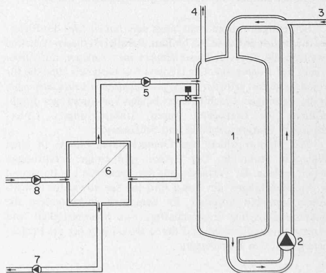
Bild 2. Prinzipschema für das aerob-thermophile Klärschlammhygienisierungsverfahren. 1 Reaktor/Fermenter, 2 Umwälzpumpe, 3 Luftabfuhr, 4 Luftzufuhr, 5 Füllpumpe, 6 Wärmetauscher, 7 Abfuhrpumpe, 8 Zubringerpumpe (Rohschlamm)
