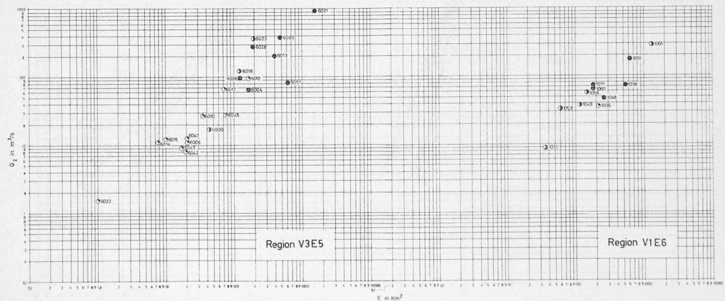
Bild 3. Alle zwei Jahre auftretendes Hochwasser Q_2 in m^3/s (Ordinate) als Funktion der Einzugsgebietsfläche E (Symbole und Legende: siehe Bild 4)
