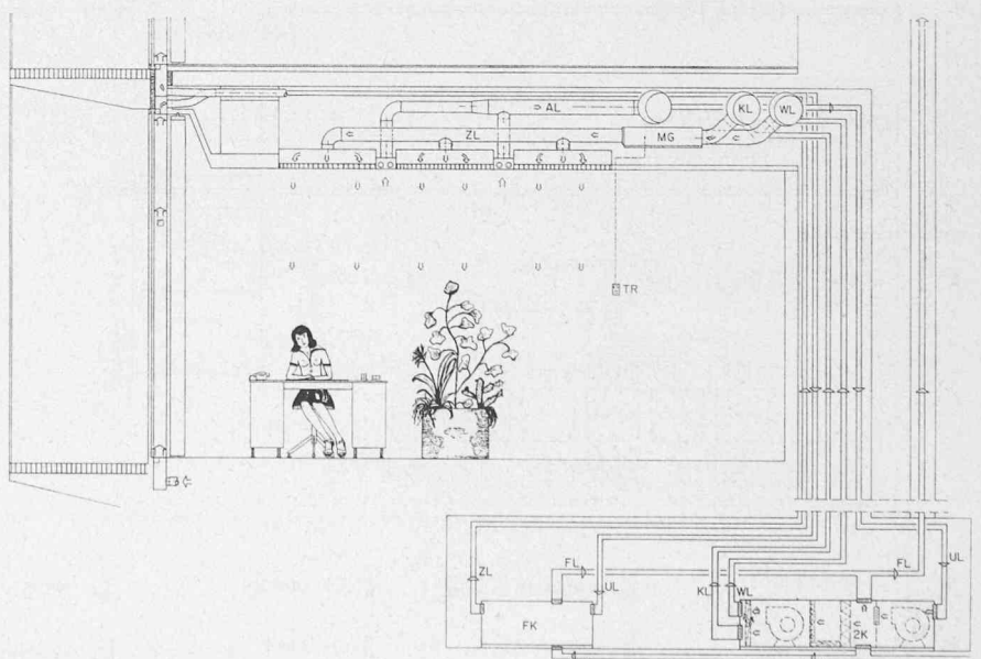
Bild 3. Lüftungsprinzip. AL Abluft, FL Fortluft, ZL Zuluft, KL Kaltluft, WL Warmluft, UL Umluft, ASL Aussenluft, TR Temperaturregler, MG Mischgerät, FK Fensterklimateur, ASL Aussenluft, 2K 2-Kanal-Klimagerät
