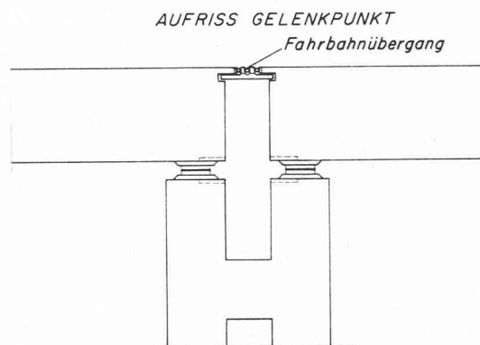
Bild 5. Detail Gelenkpunkt
