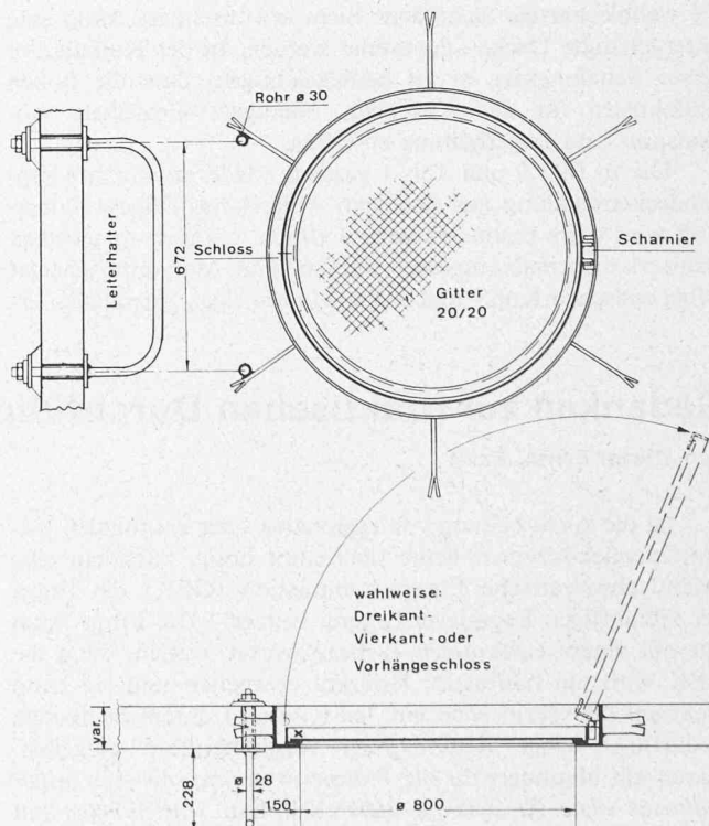
Bild 15. Hohlkasten-Einstiegluke, Hauptabmessungen
