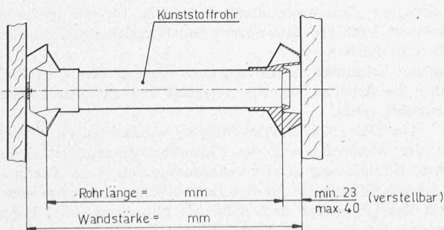
Bild 14. Futterrohr mit Haltekone
