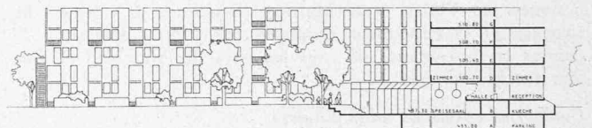
Schnitt Hotel, Ansicht von Süden 1:1000
