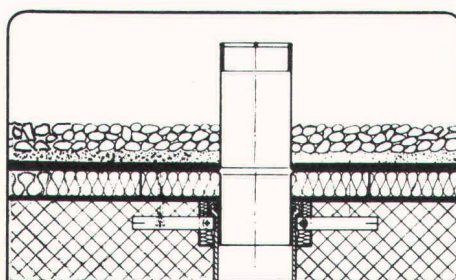
Soba-Dunstrohr Typ GS 0120
