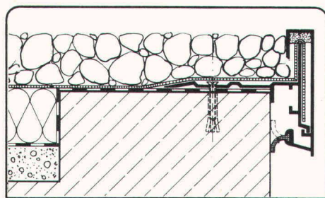
Soba-Dachrandprofil Typ GS 21 0410
