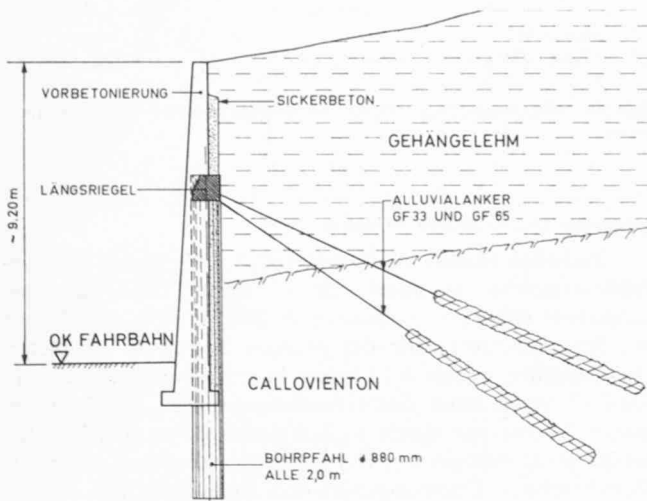
Bild 13. Stützmauer Mitteldiegtlen Süd, Nationalstrasse N 2. Abschnitt Sissach-Eptingen
