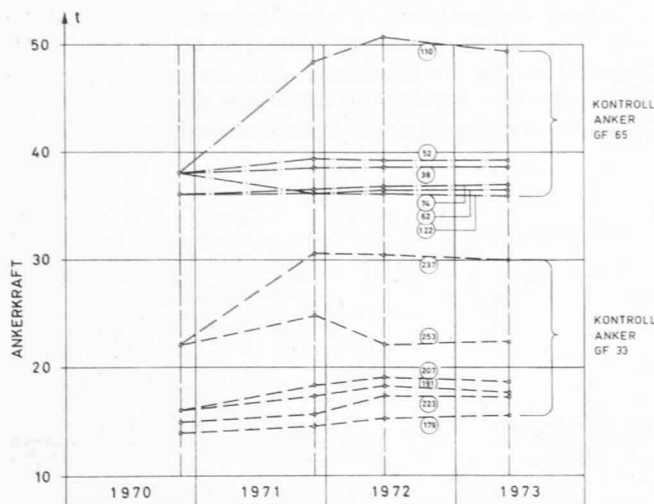
Bild 14. Kraftverlauf in den Kontrollankern Stützmauer Mitteldiegtlen, Nationalstrasse N 2
