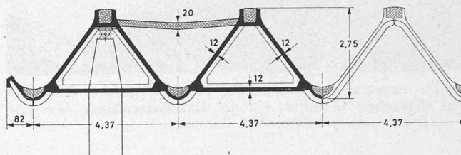
Bild 11. Paketumschlaghalle München, Querschnitt eines Stirnbogens
