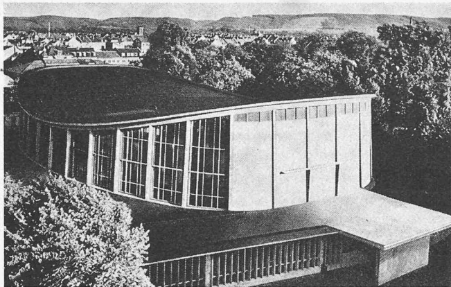
Bild 14. Schwarzwaldhalle Karlsruhe, in sich gespanntes Hängedach über elliptischem Grundriss, mit den Hauptachsenlängen 48 m und 73 m. Erstes Spannbetonhängedach Europas
