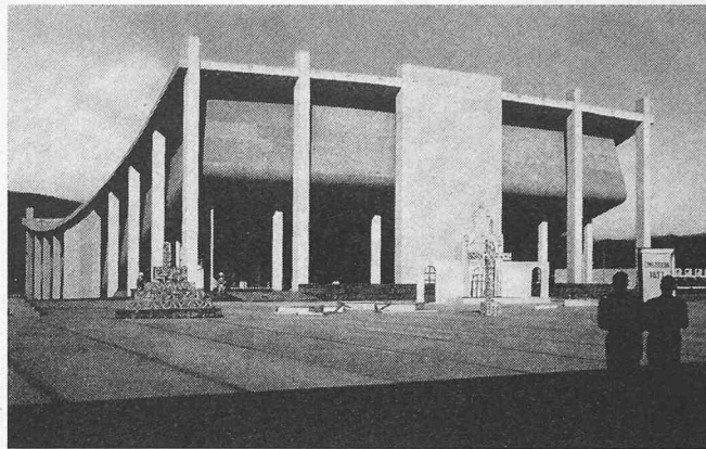
Bild 15. Auditorium Jalapa, Mexiko. In sich gespanntes Hängedach mit 71 m Spannweite über einer Grundfläche von 40 \times 71 m
