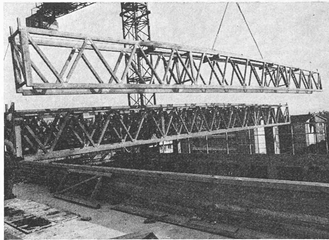
Bild 4. Montage eines Binderpaares. Die Nagelflachwerkbinder in patentierter Greimbauweise haben eine Spannweite von 26,41 m
