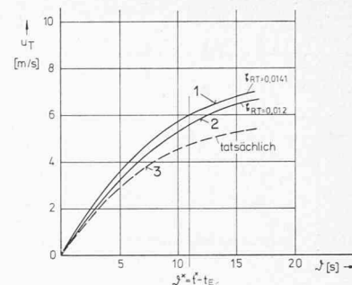
Bild 10. Tatsächlicher Geschwindigkeitsverlauf der Luftströmung im Tunnel der U-Bahn Hamburg bei Fahrt eines 4-DTW-1-Zuges in einer eingleisigen Tunnelröhre 1, 2 Rechenresultate nach Gl. [21] und [22] mit \zeta_{RT} = 0,0141 bzw. \zeta_{RT} = 0,012 3 Messergebnis
