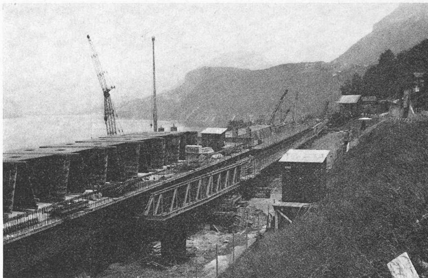
Bild 7. Vorschubgerüst nach der ersten Vorfahrt. Hinten im Bereich des betonierten Brückenfeldes der rückwärtige Fachwerk-schnabel. Dann folgt der kastenförmige Rüst-träger, der an der Koppelfuge aufgehängt ist. Vorne ist der 46 m Vorfahrschnabel mit Auf-lagerung auf der Quertraverse beim Pfeiler 4. Auf dem betonierten Teil sind 5 m lange Ele-mente der klappbaren Innenschalung zu sehen (Aufnahme: D. J. Bänziger, 21. 7. 1977)
