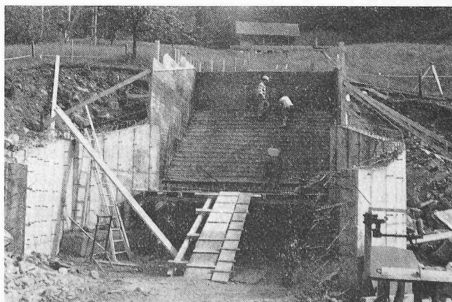
Bild 9. Erste Phase der Schachterstellung: Vom biegesteifen Schacht-ansatz (BSA) des Schachtes 14 ist hier ein segmentartiger Teil beto-niert. Bergseits wird der Schachtaufbau armiert (Aufnahme: D. J. Bänziger, 2. 6. 1977)
