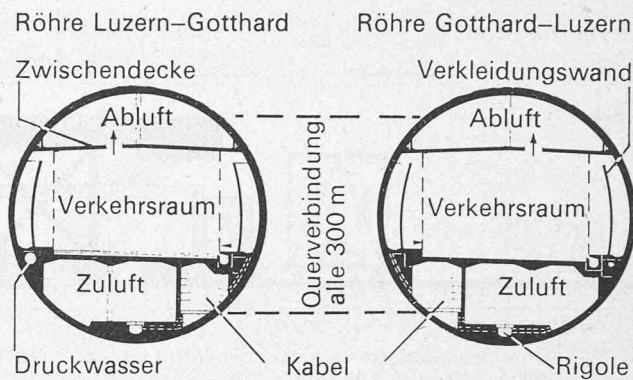
Bild 4. Kreisförmige Tunnelquerschnitte Baulos «Hutegg»
