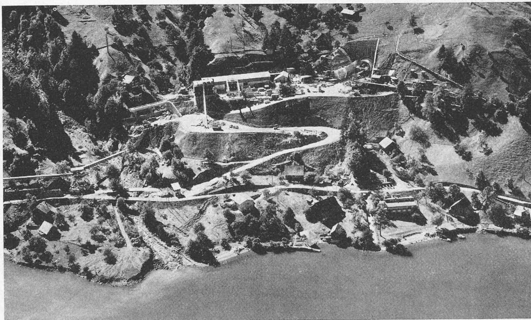
Installationsplatz der Baustelle «Huttegg». Das Bild wurde während der Erstmontage des «Big-John» aufgenommen. Es zeigt beim Lüftungstollenportal das Vorziehen des Schildes in Startposition und auf dem Tübbinglagerplatz die Montage des Baggers und des Nachläufers
