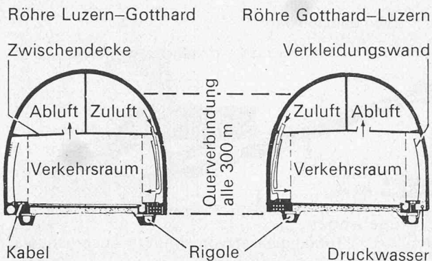
Bild 3. Hufeisenförmige Tunnelquerschnitte Baulos Nord und Baulos Süd
