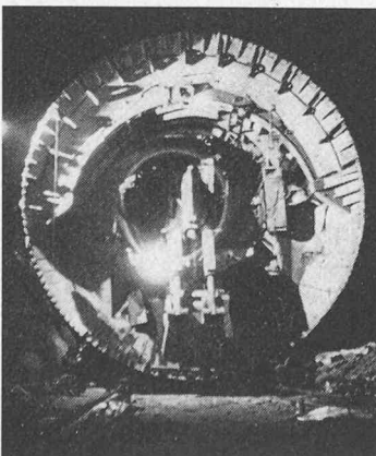
Bild 15, 16 und 17. Der Schild mit Excavator ruht auf dem Schlitten bereit zum Verschieben. Im Vordergrund die Stahlschlitten und die Verschiebebahnen (links). Der Schild während der Verschiebeaktion. Besonders gut sind in der oberen Schildhälfte die 12 Pressplatten (Messer), die einzeln ausgefahren werden können, zu erkennen (Mitte). Der Schild während des Drehens in der Bergkaverne. Unten sind der Drehtisch und der Schlitten, auf dem der Schild standfest gelagert ist, zu erkennen. Die Position des Excavators in den Führungen wurde so gewählt, dass die Wirkungslinie des Eigengewichtes der ganzen Einheit möglichst genau durchs Zentrum der Standfläche des Schlittens verlief (rechts)
