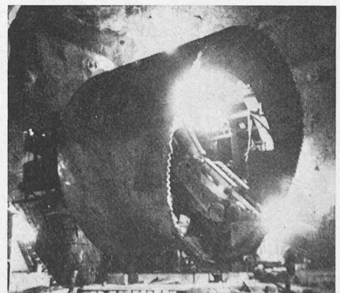
Bild 15, 16 und 17. Der Schild mit Excavator ruht auf dem Schlitten bereit zum Verschieben. Im Vordergrund die Stahlschlitten und die Verschiebebahnen (links). Der Schild während der Verschiebeaktion. Besonders gut sind in der oberen Schildhälfte die 12 Pressplatten (Messer), die einzeln ausgefahren werden können, zu erkennen (Mitte). Der Schild während des Drehens in der Bergkaverne. Unten sind der Drehtisch und der Schlitten, auf dem der Schild standfest gelagert ist, zu erkennen. Die Position des Excavators in den Führungen wurde so gewählt, dass die Wirkungslinie des Eigengewichtes der ganzen Einheit möglichst genau durchs Zentrum der Standfläche des Schlittens verlief (rechts)
