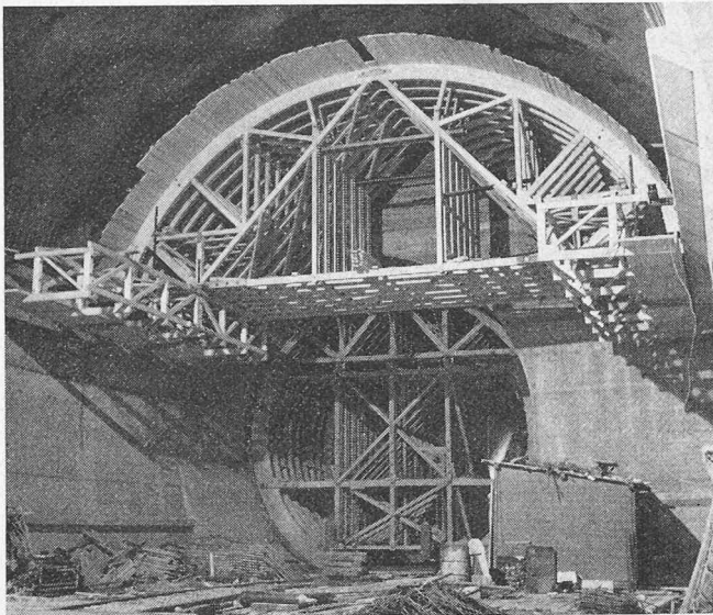
Bild 27 (links). Das Lehrgerüst steht für die erste Betonieretappe des grossen Kavernengewölbes bereit. Im Hintergrund die Starttröhrenschaalung. – Bild 30 (rechts). Auskragender Lauf- und Bedienungsteg
