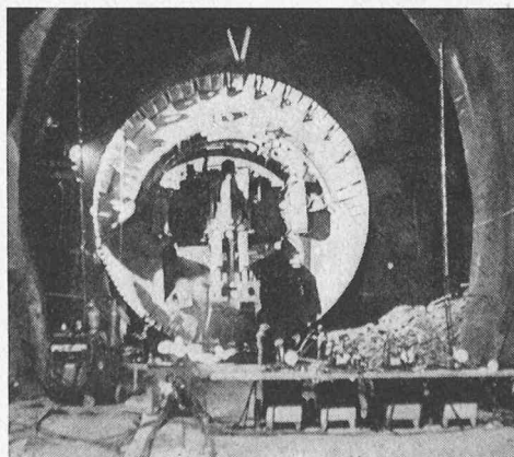
Bild 15, 16 und 17. Der Schild mit Excavator ruht auf dem Schlitten bereit zum Verschieben. Im Vordergrund die Stahlschlitten und die Verschiebebahnen (links). Der Schild während der Verschiebeaktion. Besonders gut sind in der oberen Schildhälfte die 12 Pressplatten (Messer), die einzeln ausgefahren werden können, zu erkennen (Mitte). Der Schild während des Drehens in der Bergkaverne. Unten sind der Drehtisch und der Schlitten, auf dem der Schild standfest gelagert ist, zu erkennen. Die Position des Excavators in den Führungen wurde so gewählt, dass die Wirkungslinie des Eigengewichtes der ganzen Einheit möglichst genau durchs Zentrum der Standfläche des Schlittens verlief (rechts)
