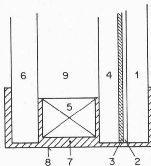
1 inneres Glas, 2 plastischer Film, 3 Heizschicht, 4 Glas, 5 Metallzwischenrahmen, 6 äusseres Glas, 7 Dichtungskitt, 8 Metallrahmen, 9 Luftzwischenraum
