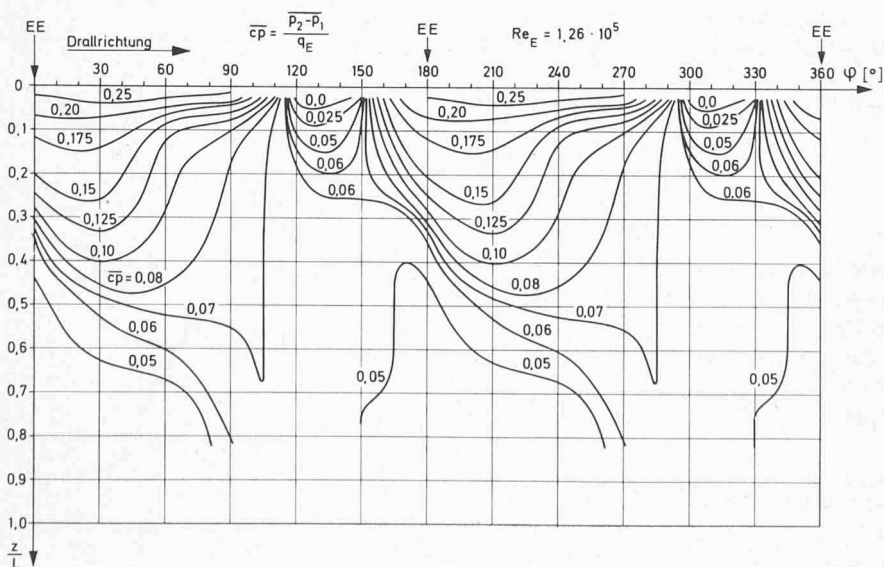
Bild 8. Verteilung der Differenz der mittleren Drücke über dem abgewinkelten Hitzeschild. (EE) Einlaufebene
