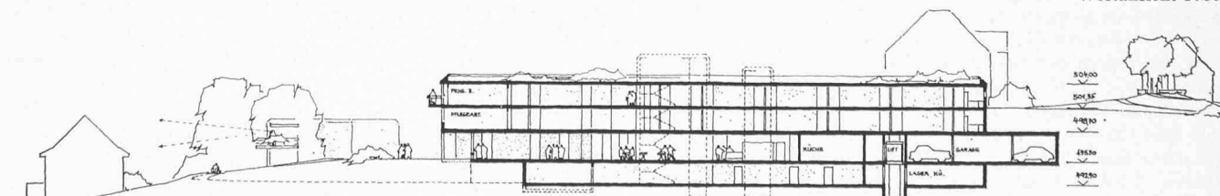
Schnitt 1:800
