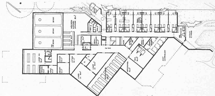
Grundriss Untergeschoss 1:800
