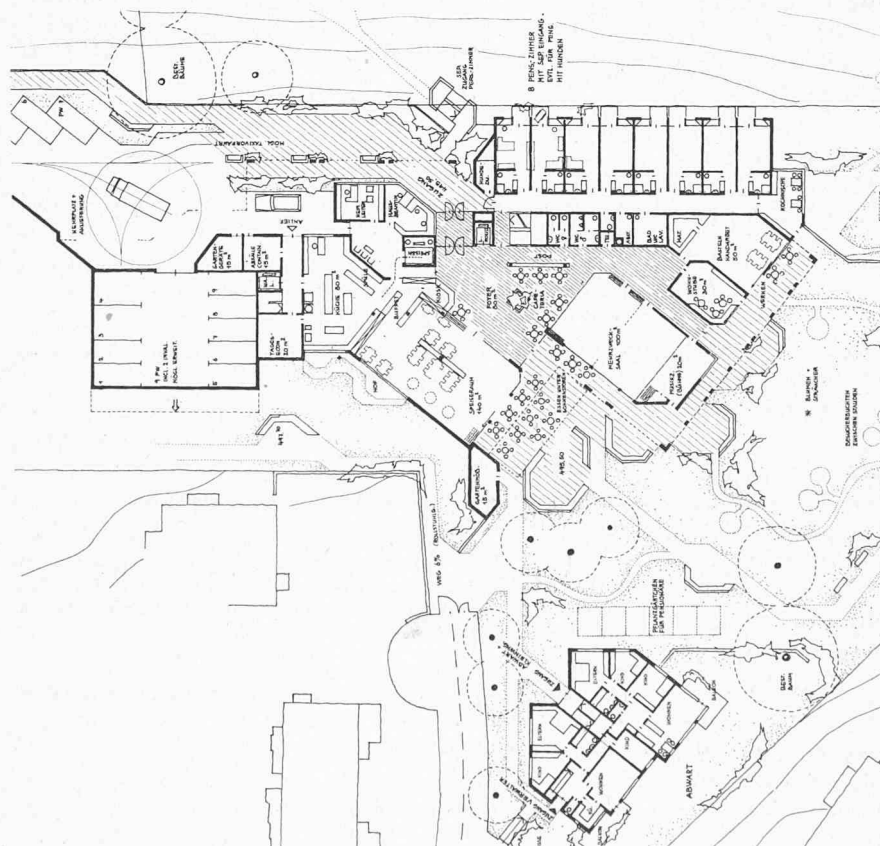
Lageplan 1:1500
