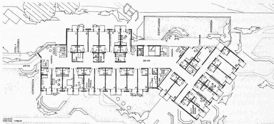
Grundriss 2. Obergeschoss 1:800
