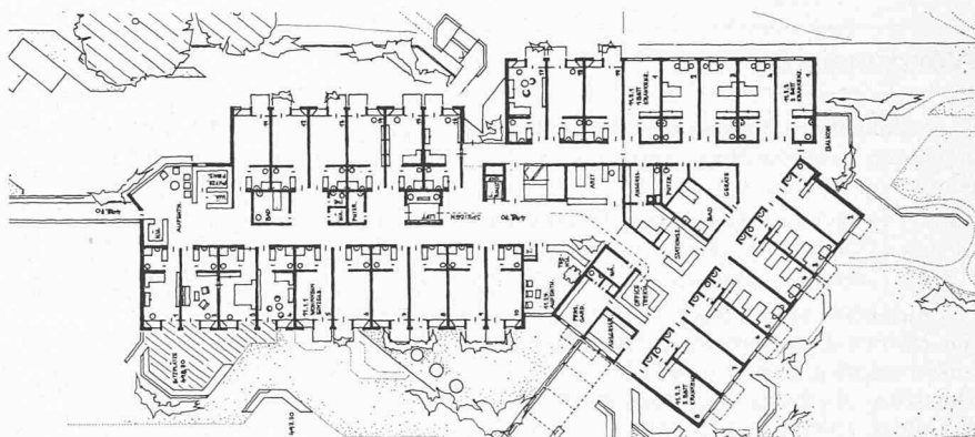
Grundriss 1. Obergeschoss 1:800
