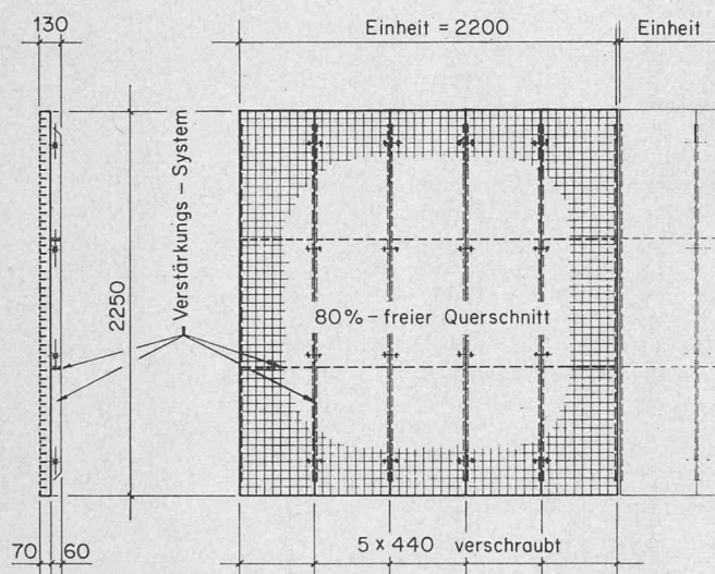
Bemessungsbeispiel. Gitterrost von hoher Tragfähigkeit ( 4,2 \text{ t/m}^2 ) ohne strömungshemmende Querträger
