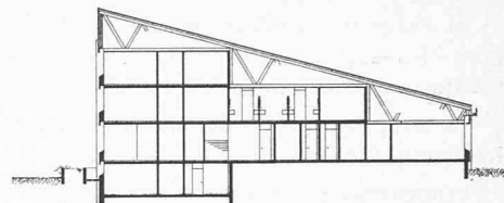
Schnitt Offiziersunterkunft 1:650
