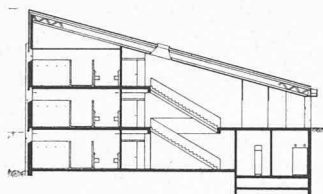
Schnitt Truppenunterkunft 1:650
