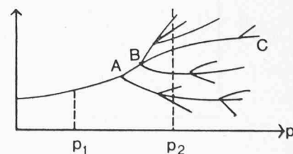
Bild 4. Gabelungsdiagramm. Lösungen
