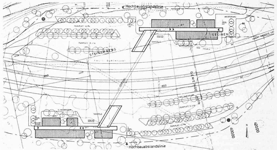
Lageplan 1:2000
