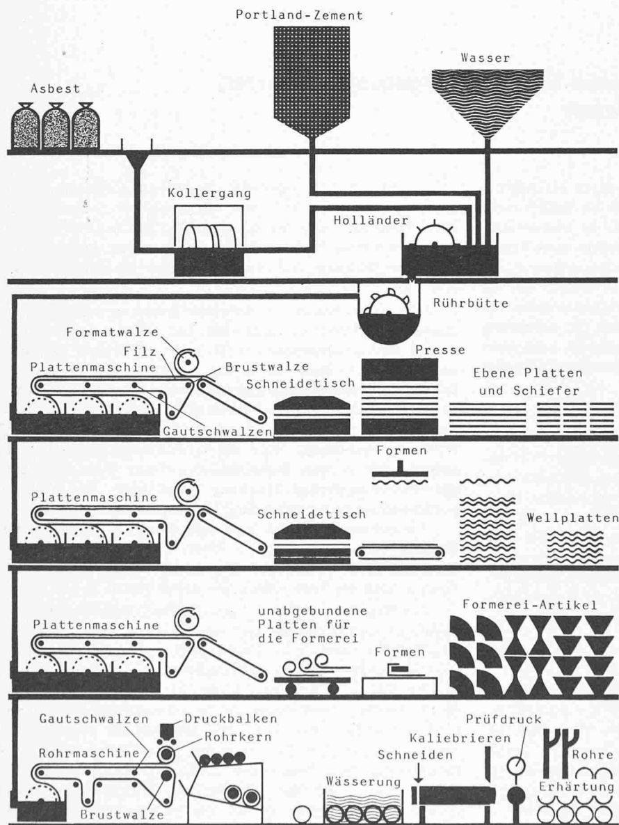
Bild 1. Fabrikationsschema
