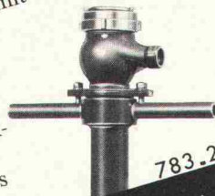
Unterflurhydrantenzähler mit Standrohr NW 25 und 50 mm (wir liefern auch Oberflurhydrantenzähler mit Storzkupplungen)
