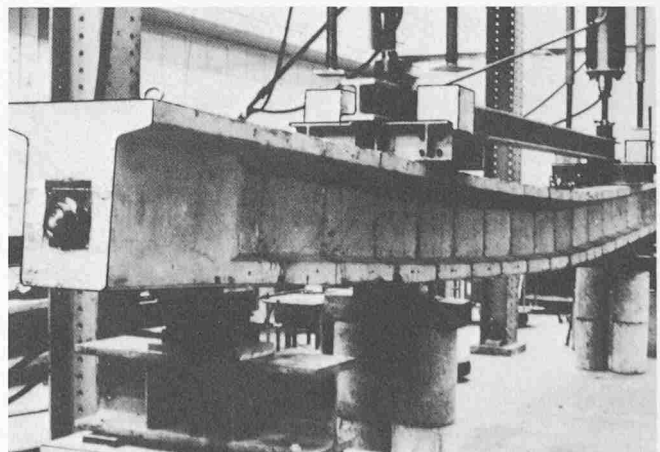
Fig. 1. Essai de poutre à voussoirs Test of segmental beam
