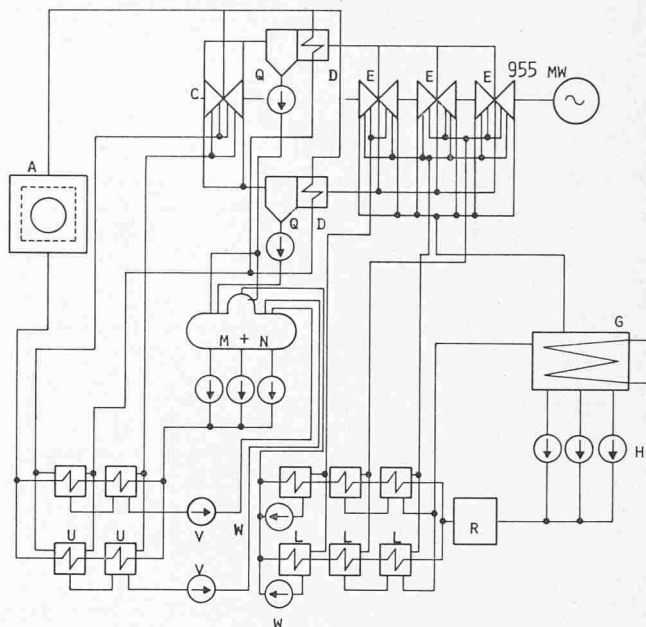
Bild 10. Kreislafschemas des Kernkraftwerkes Leibstadt
