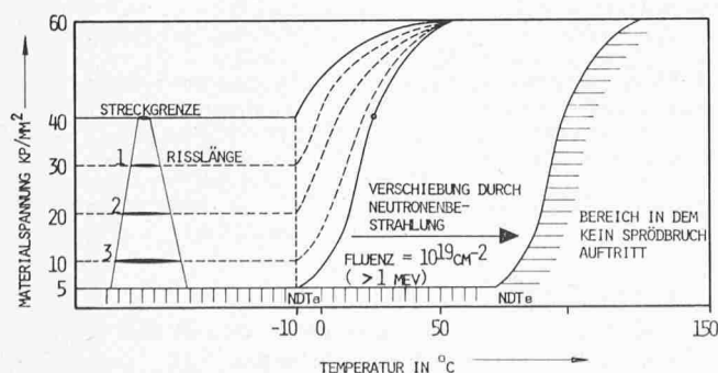
Bild 4. Erhöhung der Sprödbuchübergangstemperatur durch Neutronenbestrahlung. Sprödbuchdiagramm nach Pellini
