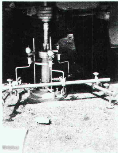
Plattenbelastungsversuch
