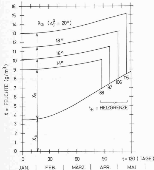
Bild 5. Zeitlicher Aufbau und Verlauf der Raumfeuchte bei k = 1,0 und d_i = 7 \text{ kcal/m}^2 \text{h } ^\circ\text{C} x_{oi} = max. zulässige Raumfeuchte x_v = max. zulässige Verdampfung x_a = Basisfeuchte (Aussenluft)
