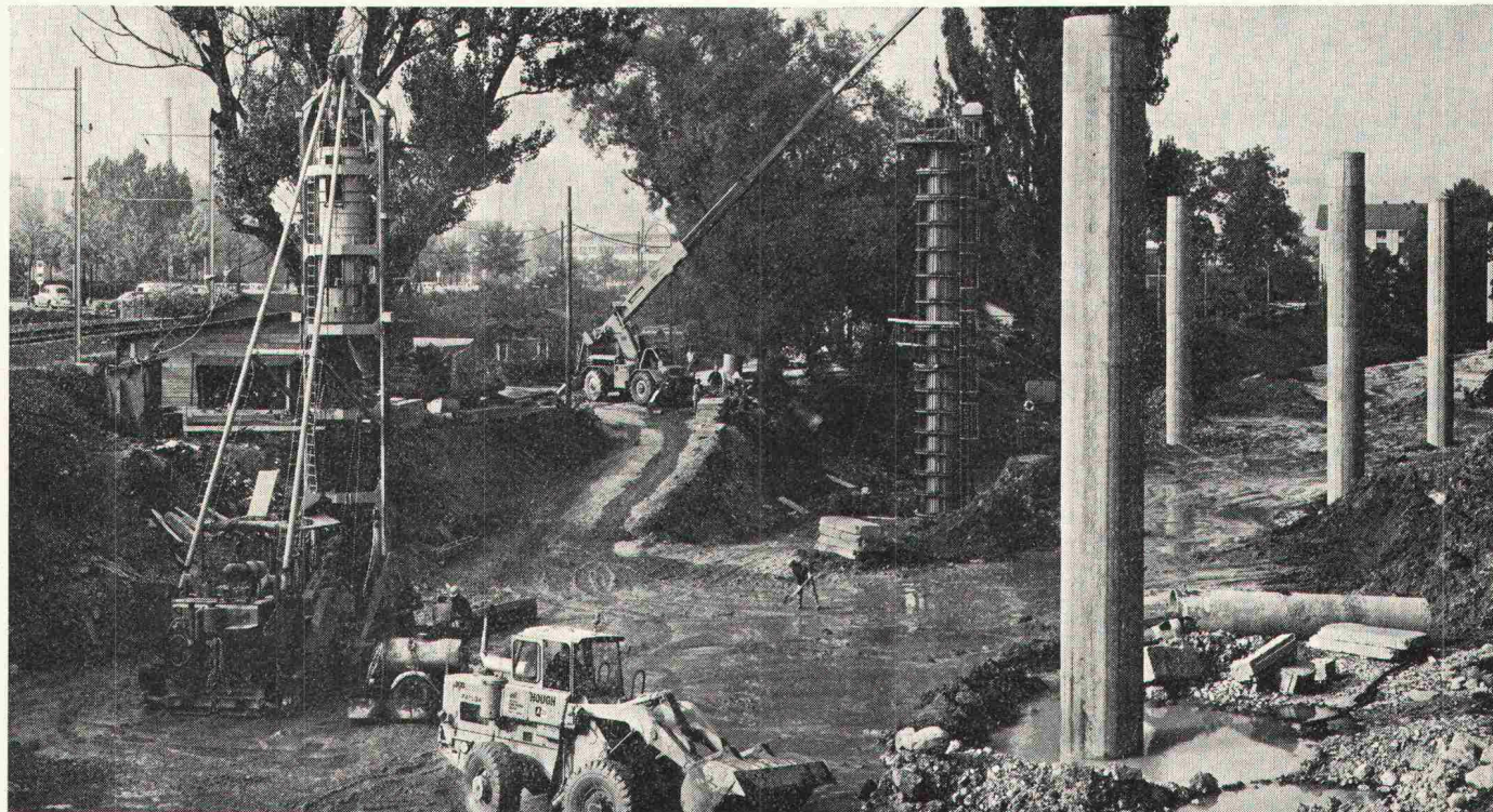
Sihlhochstrasse Zürich auf Benoto-Bohrpfählen \phi 120 und 90 cm mit Gebrauchslasten bis 640 t
