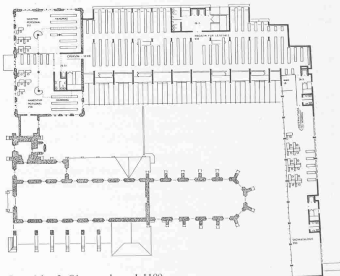
Grundriss 3. Obergeschoss 1:1100
