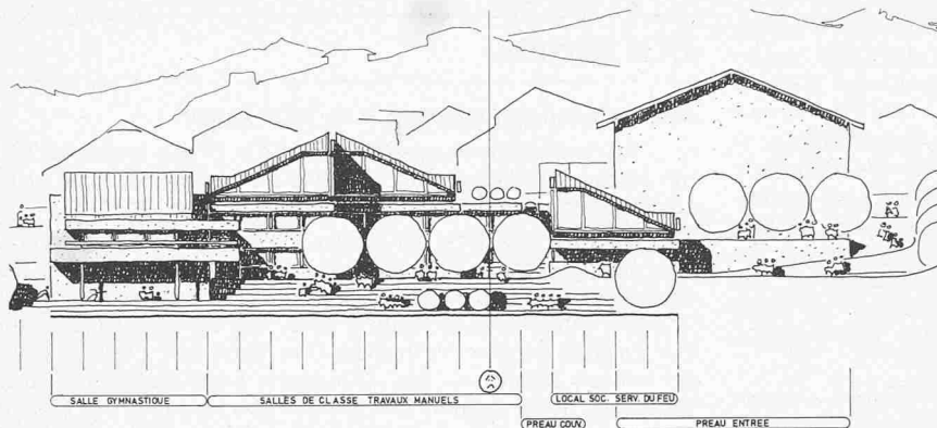
Ansicht von Süden 1:700, links Turnhalle, rechts bestehendes Schulhaus
