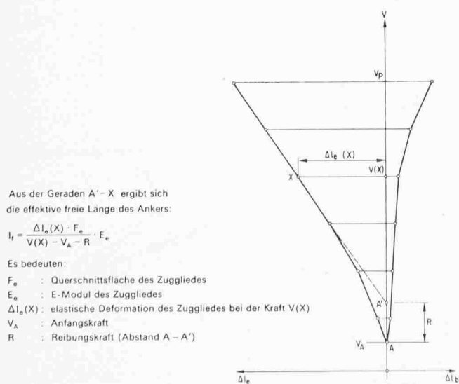
Bild 10. Diagramm der elastischen und bleibenden Deformation
