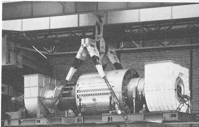
Bild 8. Sulzer Gasturbine Typ 7, mit N_{CI MAC} \approx 10000 kW
