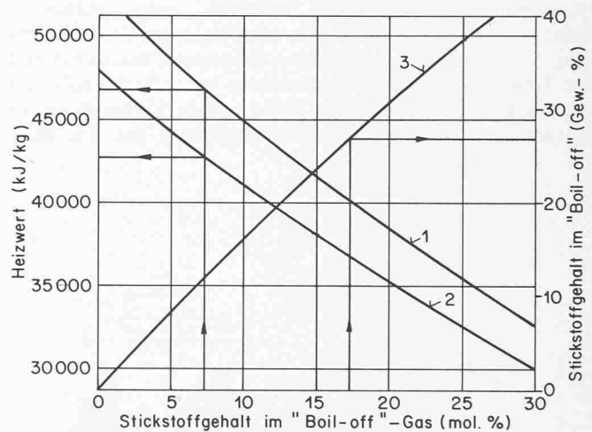
Bild 5. Heizwert des «boil-off» ( H_o \text{ Methan} = 55515 \text{ kJ/kg} , H_u \text{ Methan} = 50000 \text{ kJ/kg} ). 1 Oberer Heizwert, 2 Unterer Heizwert, 3 Stickstoffgehalt
