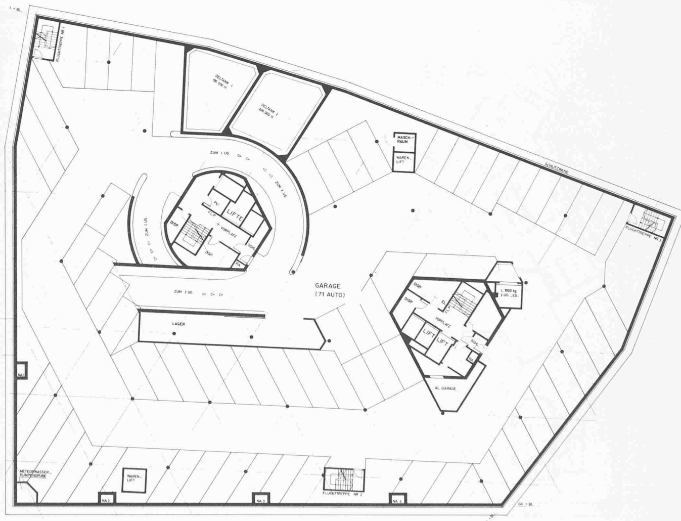
Grundriss 2. Untergeschoss 1:400
