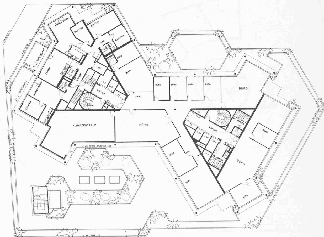
Grundriss 2. Obergeschoss 1:400
