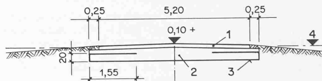
Normalprofil einer Strasse in der Umgebung Amsterdams, wo Gewebe als Hüllmaterial verwendet wurde. 1,8 cm Kiessand asphaltbeton, 2,40 cm poröse Schlacke 0-300, 3 Nicol-Stabilitätsgewebe, 4 Amsterdamer Pegel
