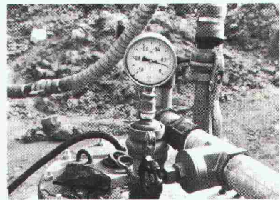
Wasserhaltung mit Vakuumbrunnen
