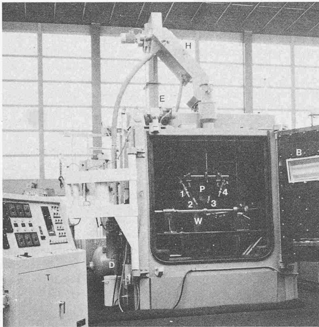
Bild 16. Nach dem Druckluft-System arbeitende, mit insgesamt fünf verstellbaren Injektorstrahlpistolen ausgerüstete Shot-peening-Kabine. Strahlmittelzuführung mit Becherwerk nach Gravitationssystem. Schaltpult mit Programmvorwahl für alle wesentlichen Parameter. W zu behandelnde Nockenwelle, E Becherwerk, H Kaskadenabscheider, B Beleuchtungseinrichtung, T Schaltpult mit Programmvorwahl für Strahlzeit, Bewegungsabläufe der Düsenköpfe usw., P Injektorstrahlpistolen: No. 1 und No. 4 führen Translationsbewegung entlang der Welle aus, No. 2 und No. 3 sind stationär auf die Seitenflächen der Nocken ausgerichtet, D zentraler Druckluftbehälter (Werkphoto: Société Bugatti S.A., Molsheim)
