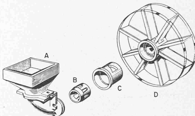
Bild 2. Die hauptsächlichen Bauelemente des von Minich 1934/35 in USA patentierten Schleuderrades mit indirekter Einführung des Strahlmittels durch mechanische Vorbeschleunigung mit Hilfe von Einlaufstück und Verteiler (s. auch Bild 1)
