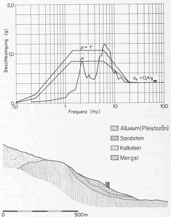
Bild 19. Lokaleinflüsse. Ermitteltes Verhaltensspektrum der Station Cornino-Forgania (Friaul, 6. Mai 1976) im Vergleich mit einem Bemessungsspektrum nach Newmark (unten). Deutlich kommt der spezifische Lokaleinfluss im Vergleich zum gemittelten Verhaltensspektrum zum Ausdruck
