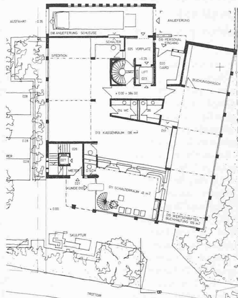
Grundriss Erdgeschoss 1:450
