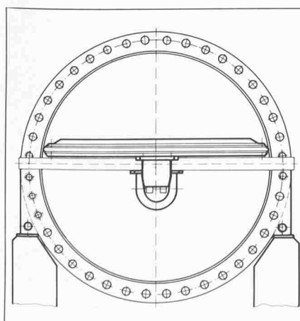
Bild 3. Schwenklappe. 1 Drehteller, 2 Querträger, 3 Abstützung, 4 Servomotor, 1 + 5 Strömungskörper
