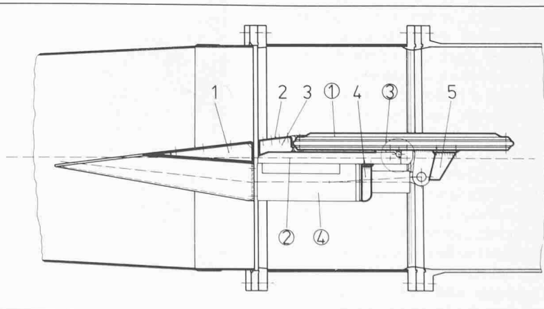
Bild 3. Schwenklappe. 1 Drehteller, 2 Querträger, 3 Abstützung, 4 Servomotor, 1 + 5 Strömungskörper
