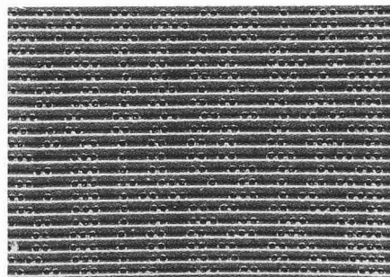
Bild 4. Mit dem Elektronenstrahlmikroskop angefertigtes Bild. Es zeigt die in die Speicherplatte eingepreßten Spuren
