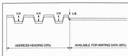
Bild 3. Längsschnitt durch die vorgeprägte Rille, in welche die Daten geschrieben werden. Den Beginn eines Sektors markiert ein Adressvorspann, dessen geprägte Daten eine Höhe von einem Viertel der Wellenlänge haben
