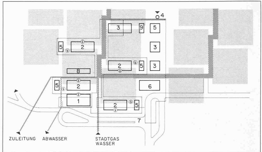
Übersicht Medienererschliessung 1. Etappe. 1 Sanitär Rayonzentrale, 2 Gebäudezentrale, Wärme und Lüftung, 3 Klimazentrale, Hörsäle bzw. EDV, 4 Stollen mit Dampfzuleitung und Telefon, 5 Elektrisch Transformatoren, 6 Kältezentrale, 7 Vorfahrt Güterumschlag, 8 Notstromversorgung, 9 Telefonverteilstation.
