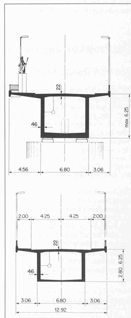
Bild 5. Querschnitte
